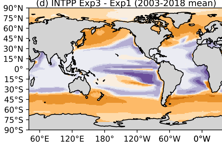
(d) INTPP Exp3 - Exp1 (2003-2018 mean)
