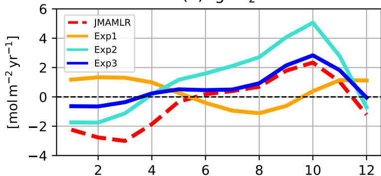
(c) DIC
