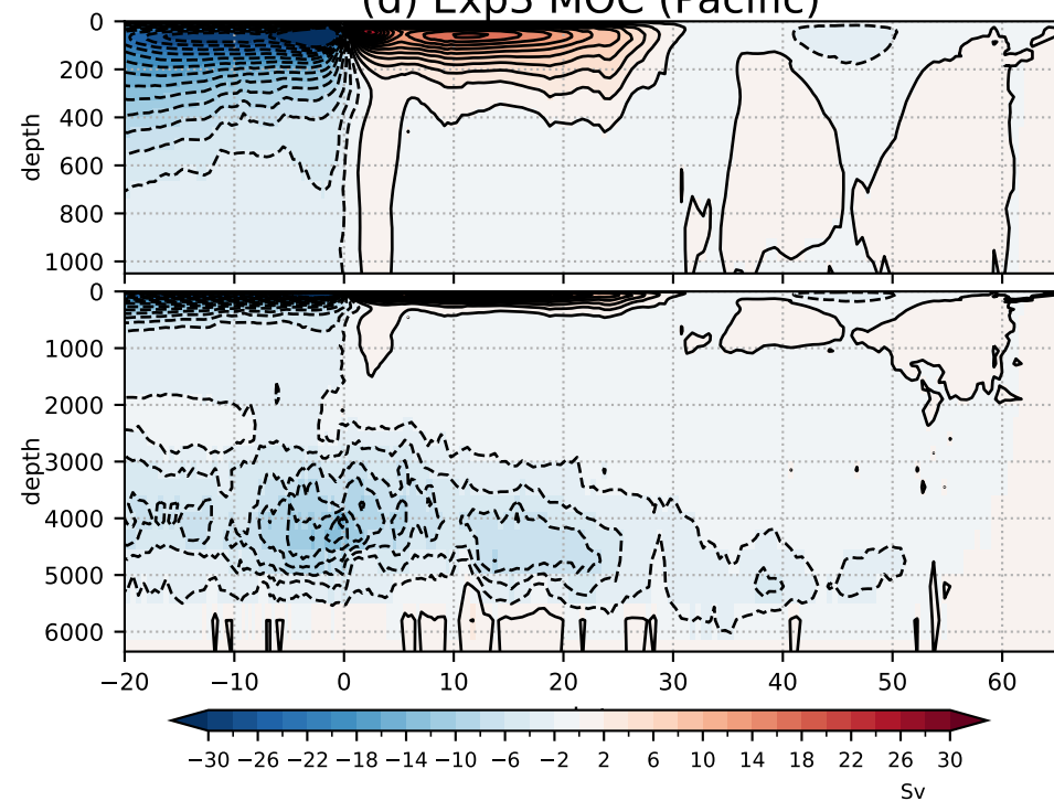
(d) Exp3 MOC (Pacific)
